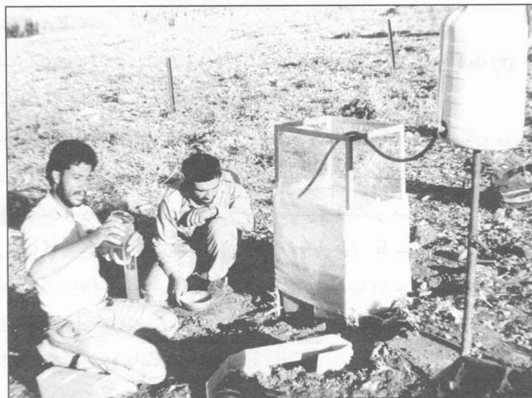
شکل ۲- نفوذسنج باران ساز و پلات آزمایشی
