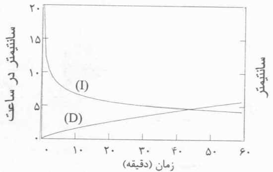
شکل ۴- نمایش منحنی‌های سرعت نفوذ لحظه‌ای (I) و نفوذ تجمعی (D) در وضعیت‌های قرق و چرا در تپه‌های گیاهی ۱، ۲، ۳ و ۴ (ب)
